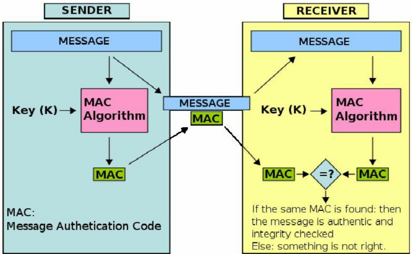
MAC的防篡改原理图
