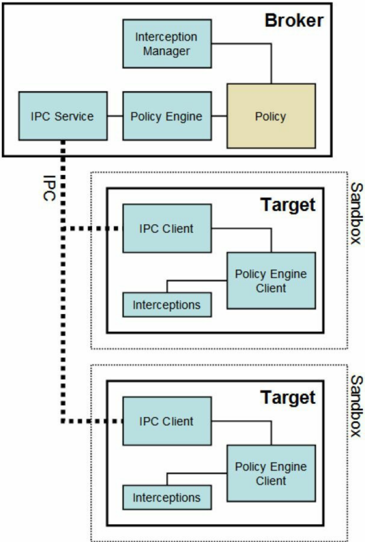
Google Chrome的Sandbox架构
